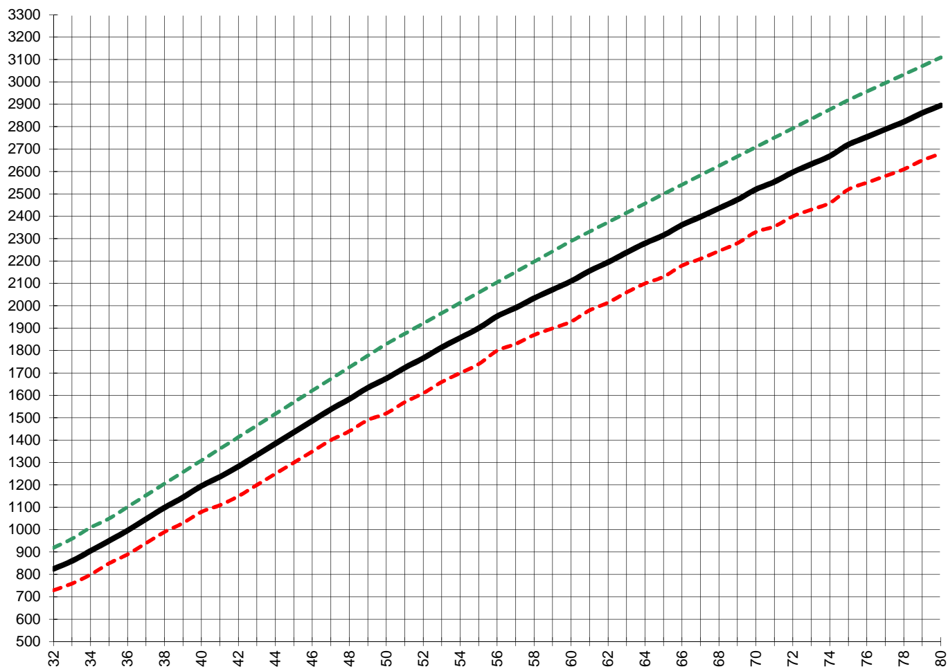
Curva de crecimiento teórica del producto terminal HYLA
